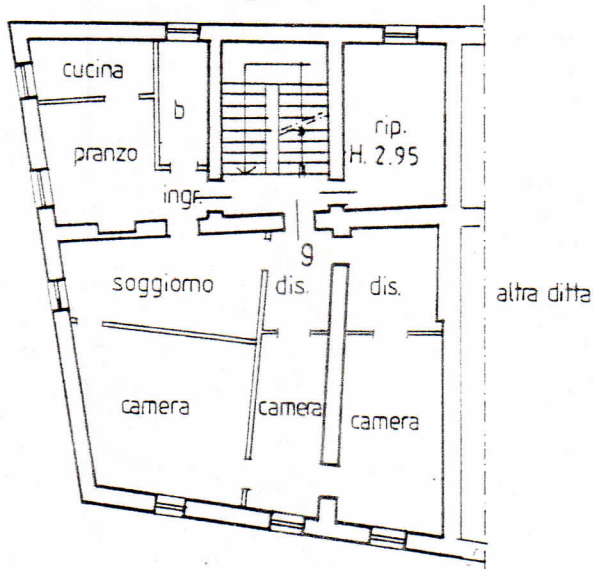
PIANO PRIMO H. 3.00
