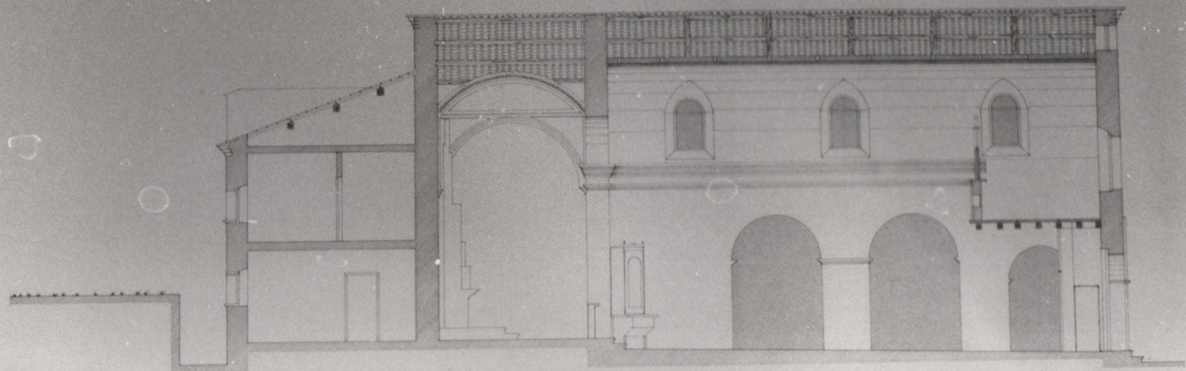
Morano C. SEZIONE SULLA CHIESA (LONGITUDINALE) Convento dei Cappuccini 0 1 2 3 4
