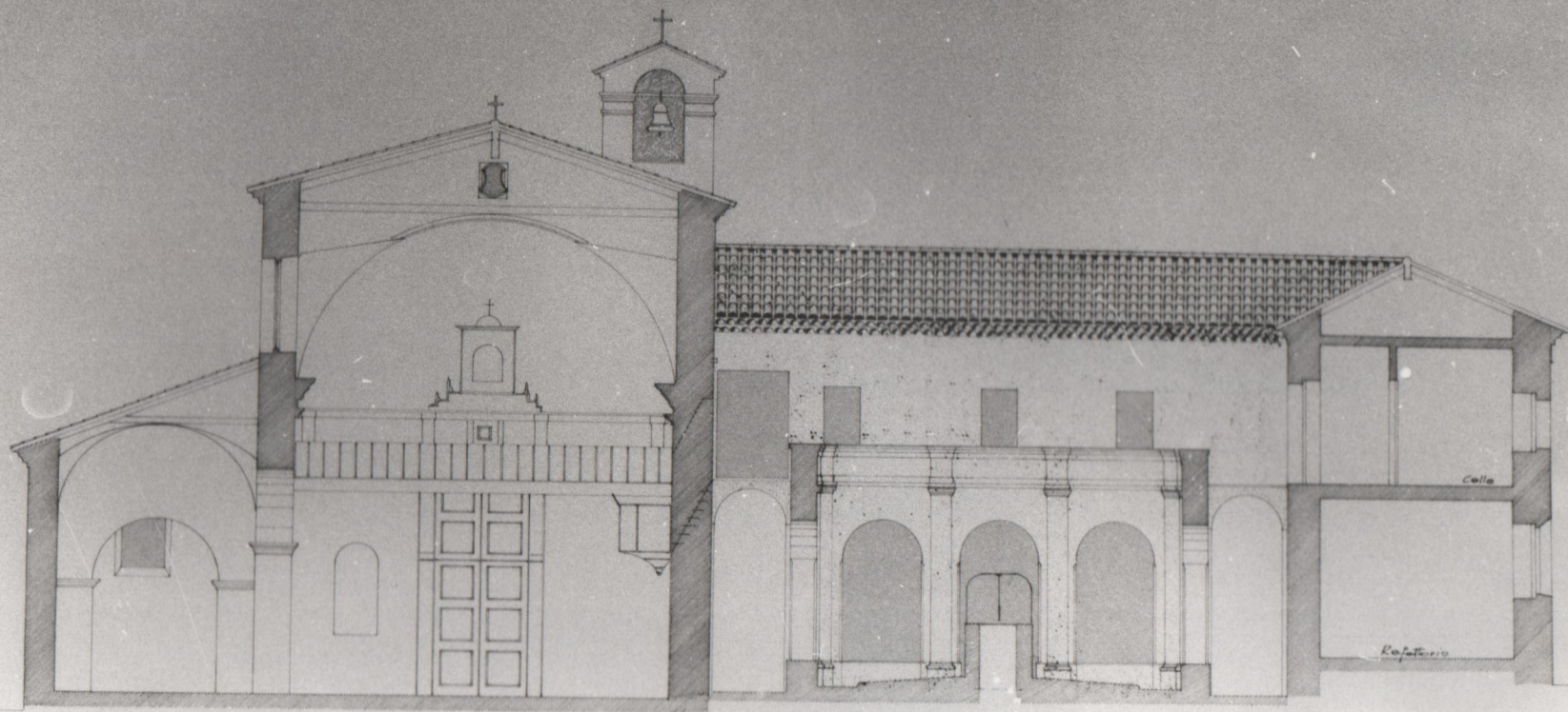
SEZIONE SUL CHIOSTRO (TRASVERSALE)
