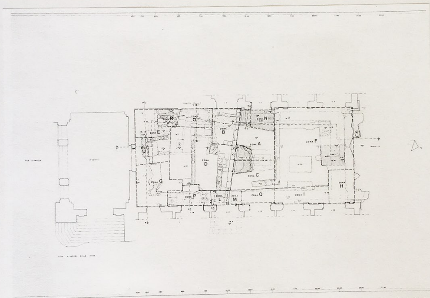
Rilievo archeologico. Pianta del livello al di sotto del solaio di calpestio della navata. Il rilievo è stato redatto dalla Soprintendenza Archeologica
