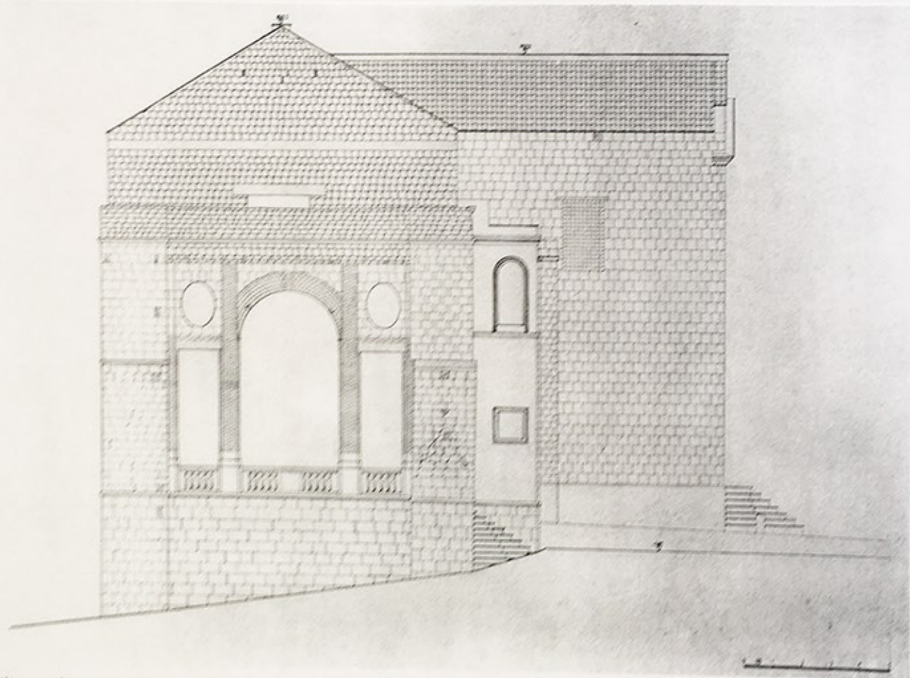
Rilievo architettonico. Prospetto della chiesa su vico S. Aniello; sono evidenti gli effetti degli impianti di consolidamento effettuati sui muri perimetrali
