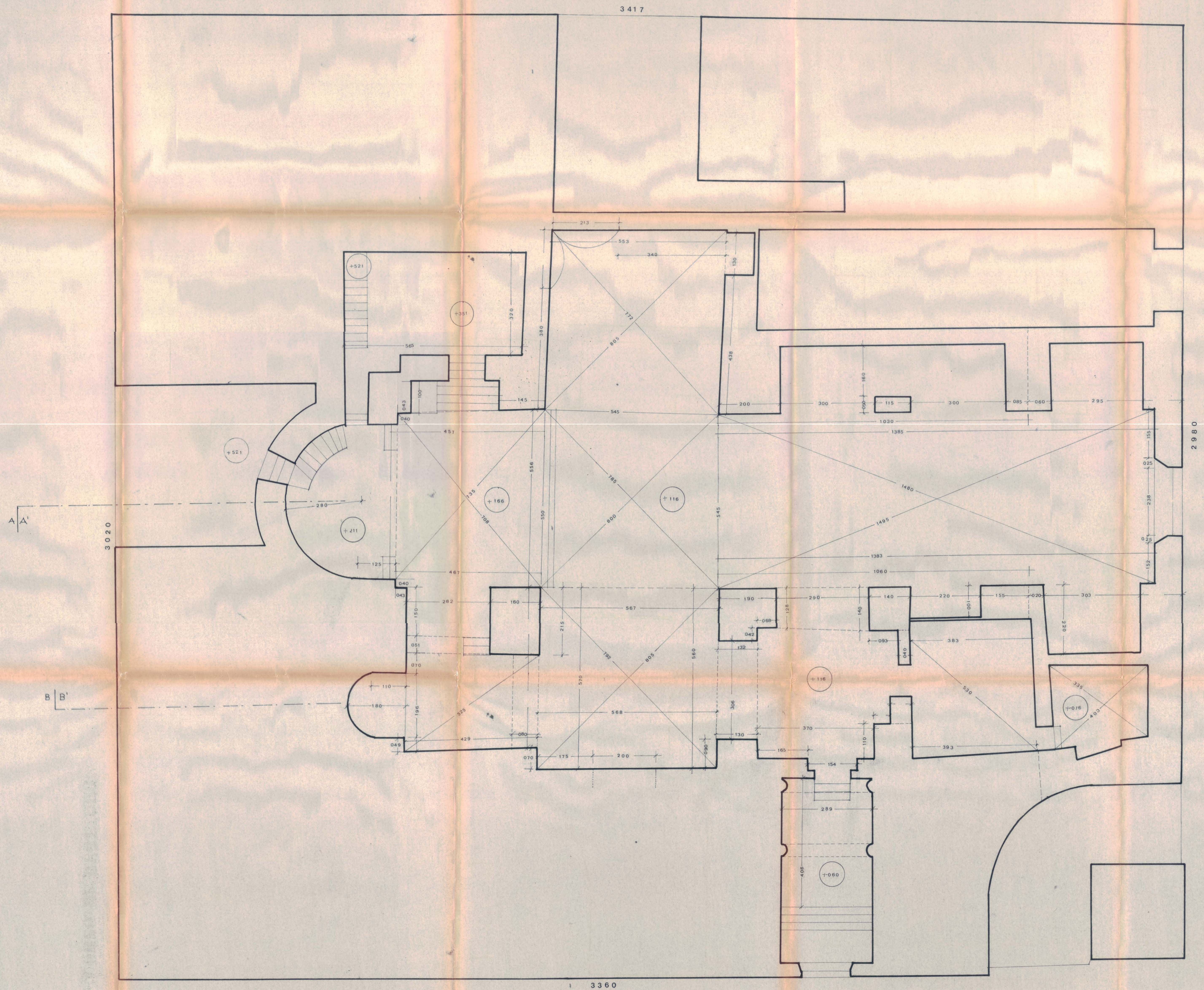
CHIESA DI S. ANTIOCO PIANTA QUOTATA RAPP. 1:50
