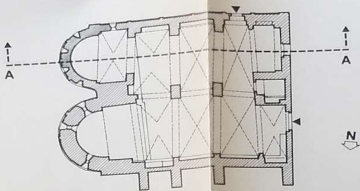
PIANTA SCHEMATICA SCALA 1/200
