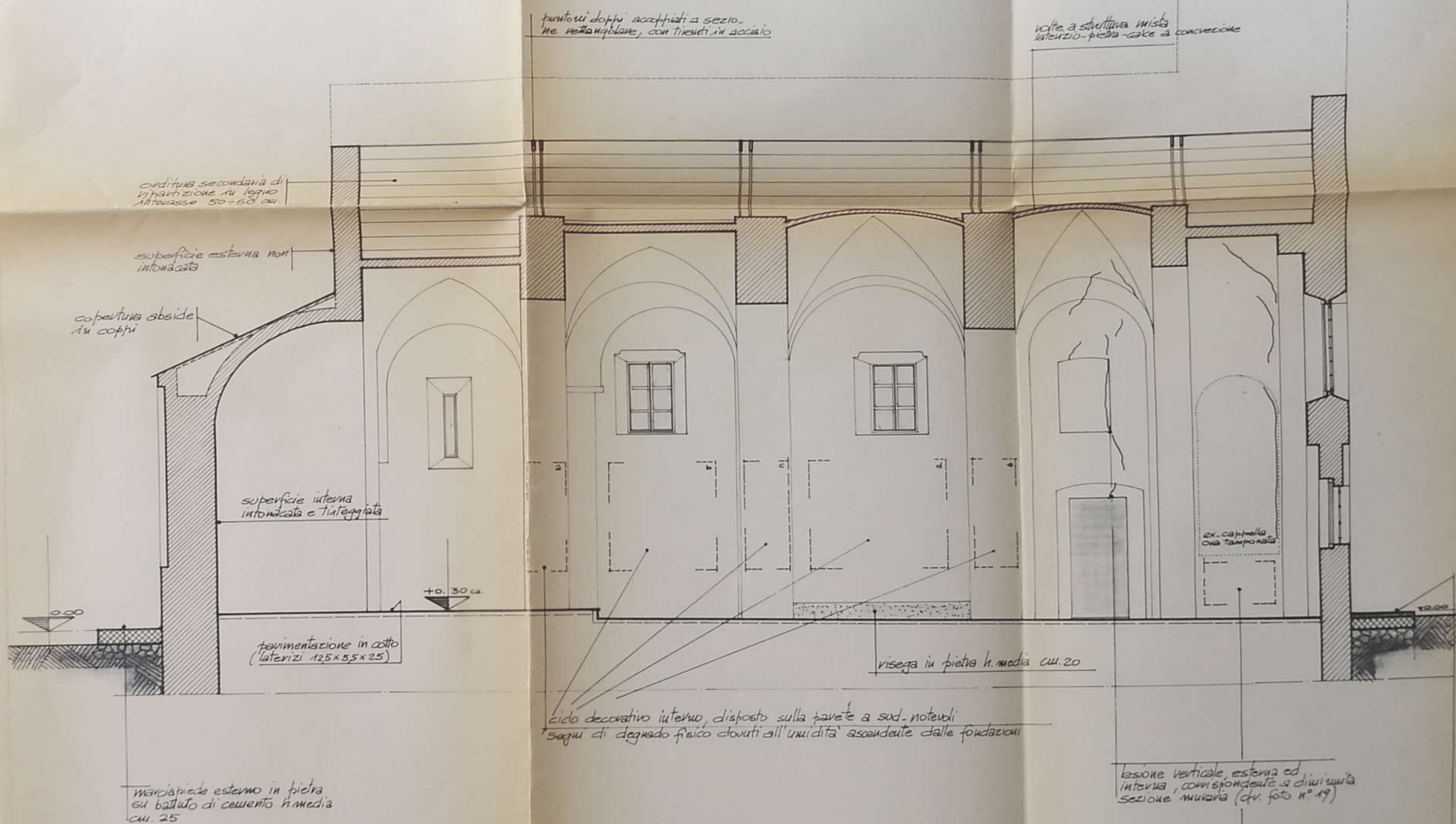
SEZIONE LONGITUDINALE AA
