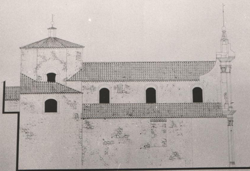
CHIESA DI S. MARINA V. CASOLE B. - PROSPETTO NORD
