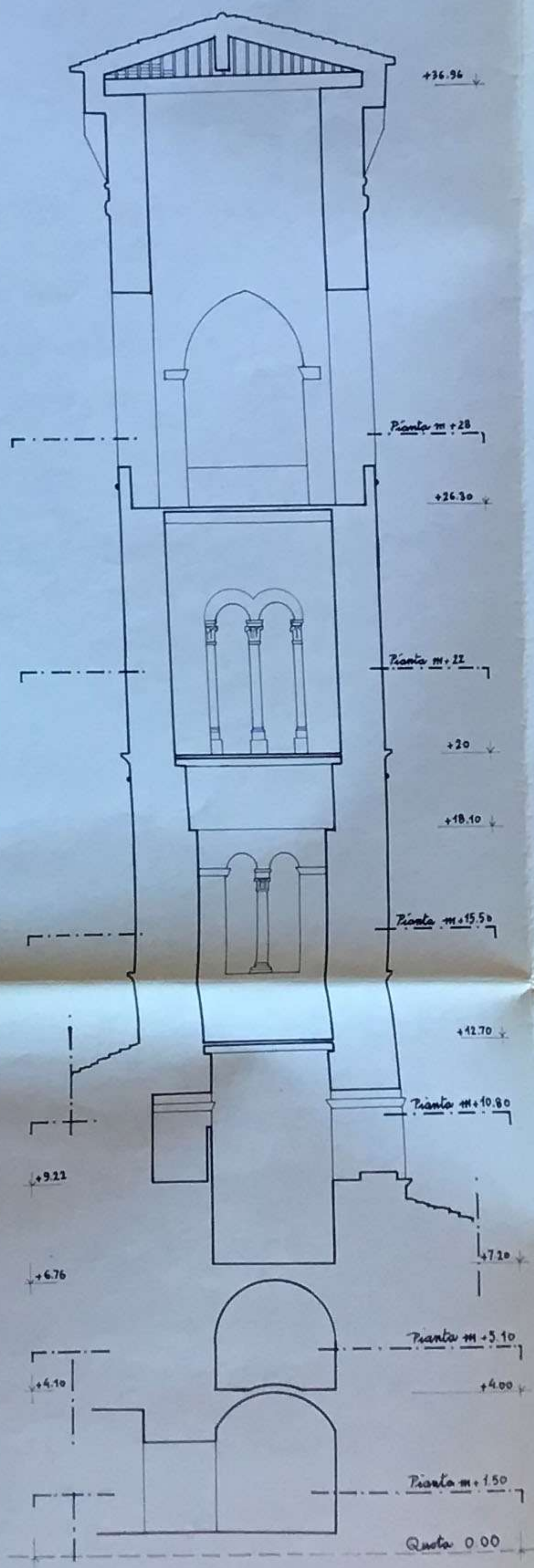
Sezione AA' Scala 1:100
