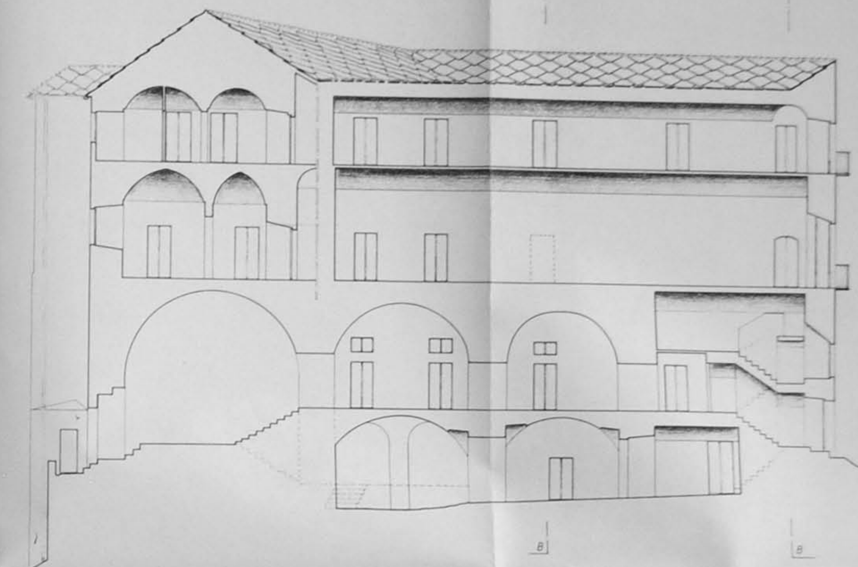
sezione CC
