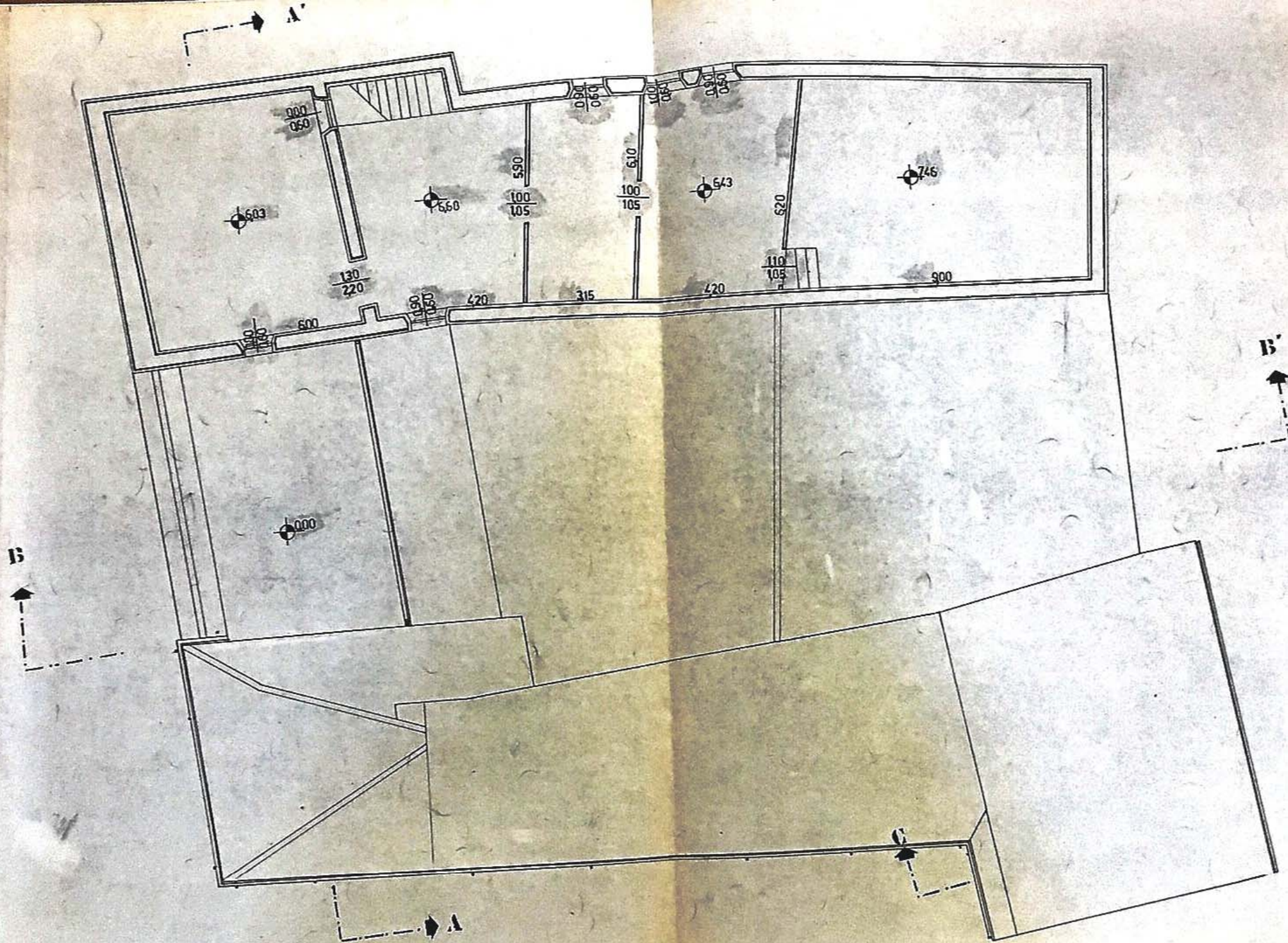
PIANTA DEL PIANO SOTTOTETTO A Q.6.68 RAPP.1.00
