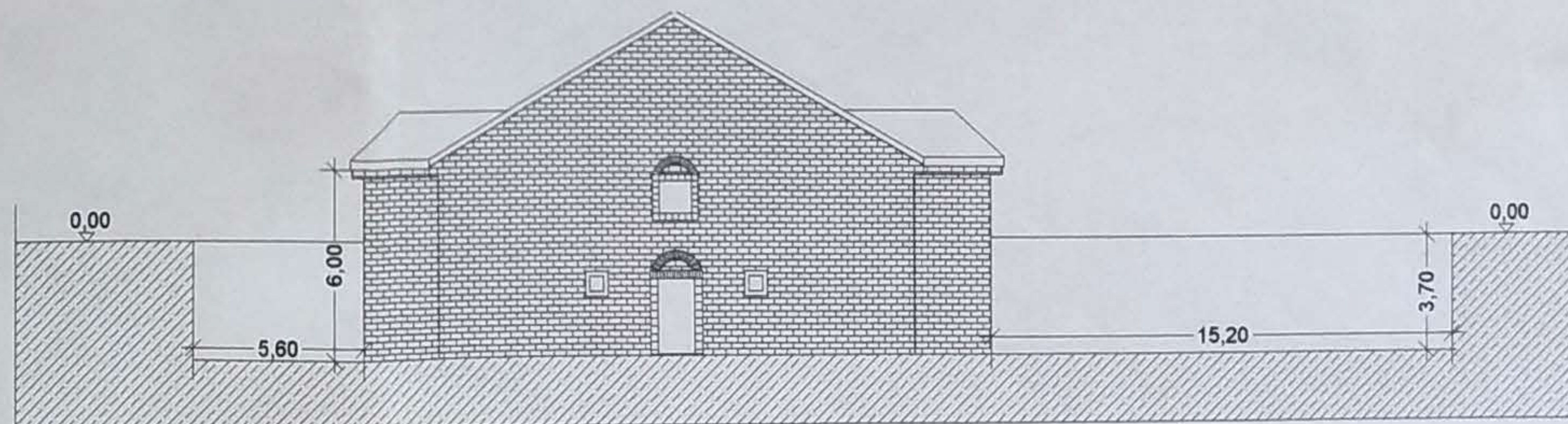
PROSPETTO NORD-OVEST
