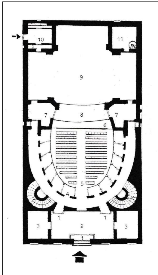
IPOTESI PIANTE REAL TEATRO SAN FERDINANDO da Antonio Iezzi, Dal Real Teatro San Ferdinando al Teatro Marrucino , eDICOLO editrice, (a cura del) Comune di Chieti – Istituzione Deputazione Teatrale Teatro Marrucino, nota introduttiva di Gabriele Obletter “Le strutture antiche”, Chieti 1997
