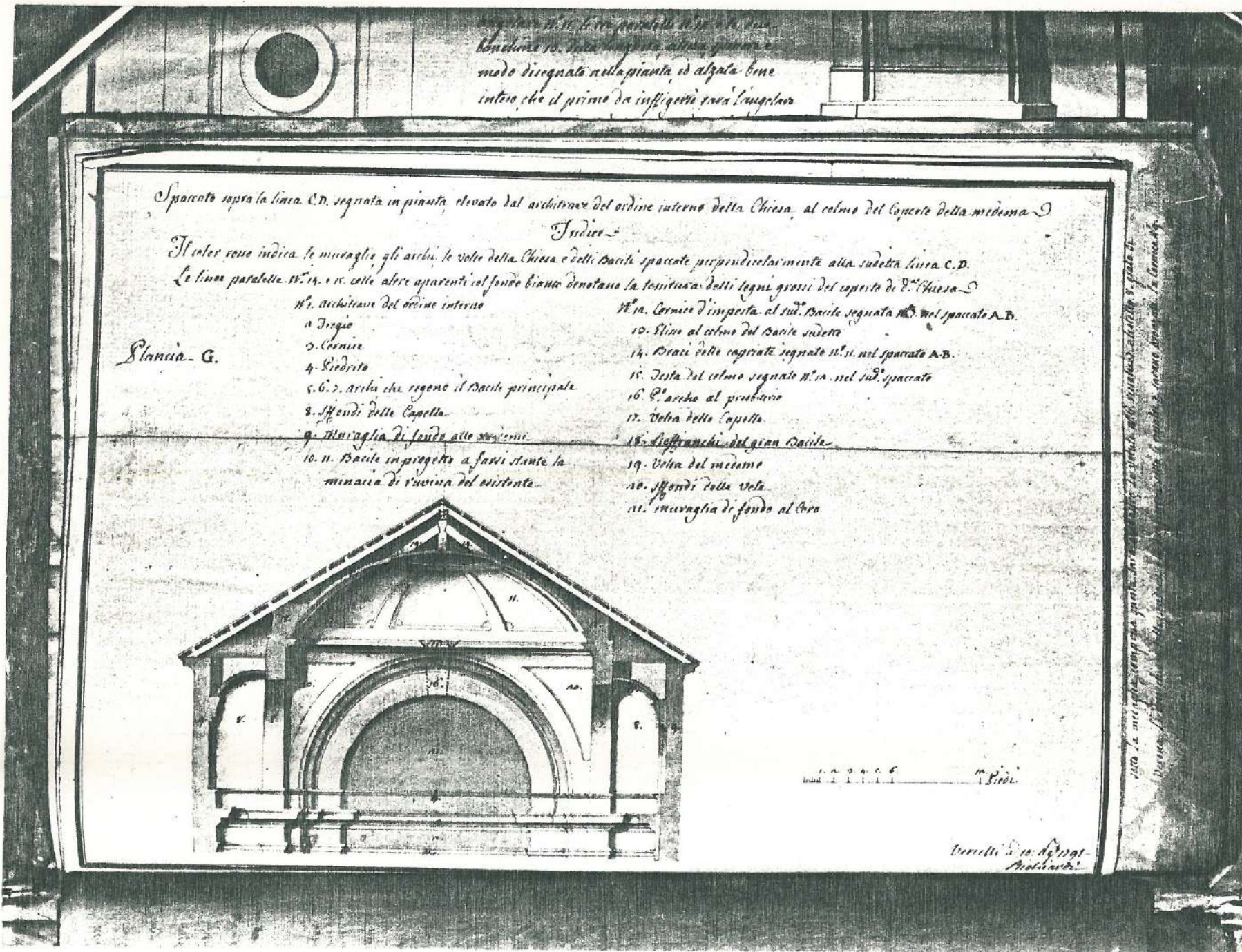
Michele Richiardi: sezione della cupola di S. Lorenzo, 1791, A.O.T.
