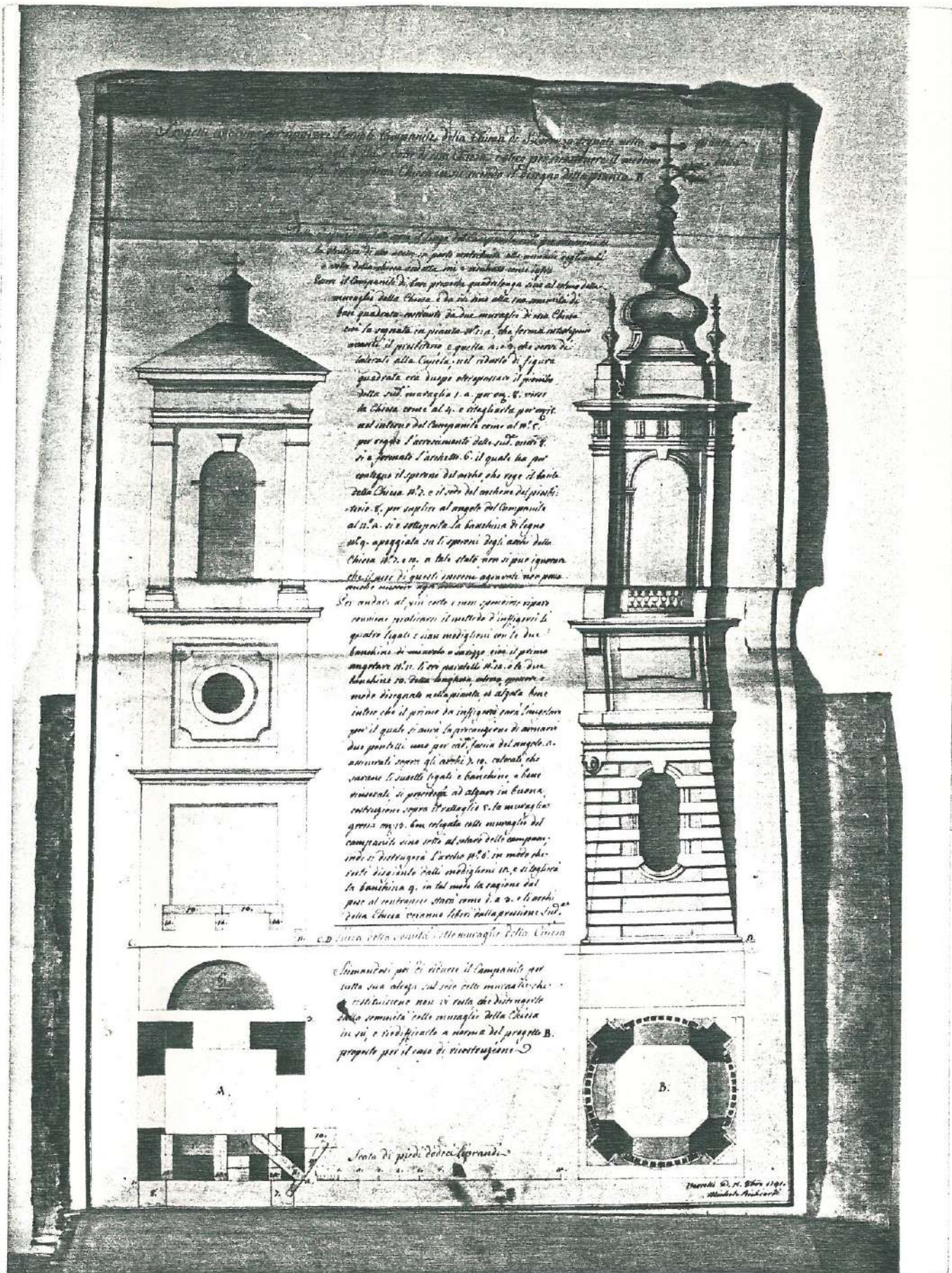
Michele Richiardi: Progetto per il campanile di S.Lorenzo, 1791, A.O.T.
