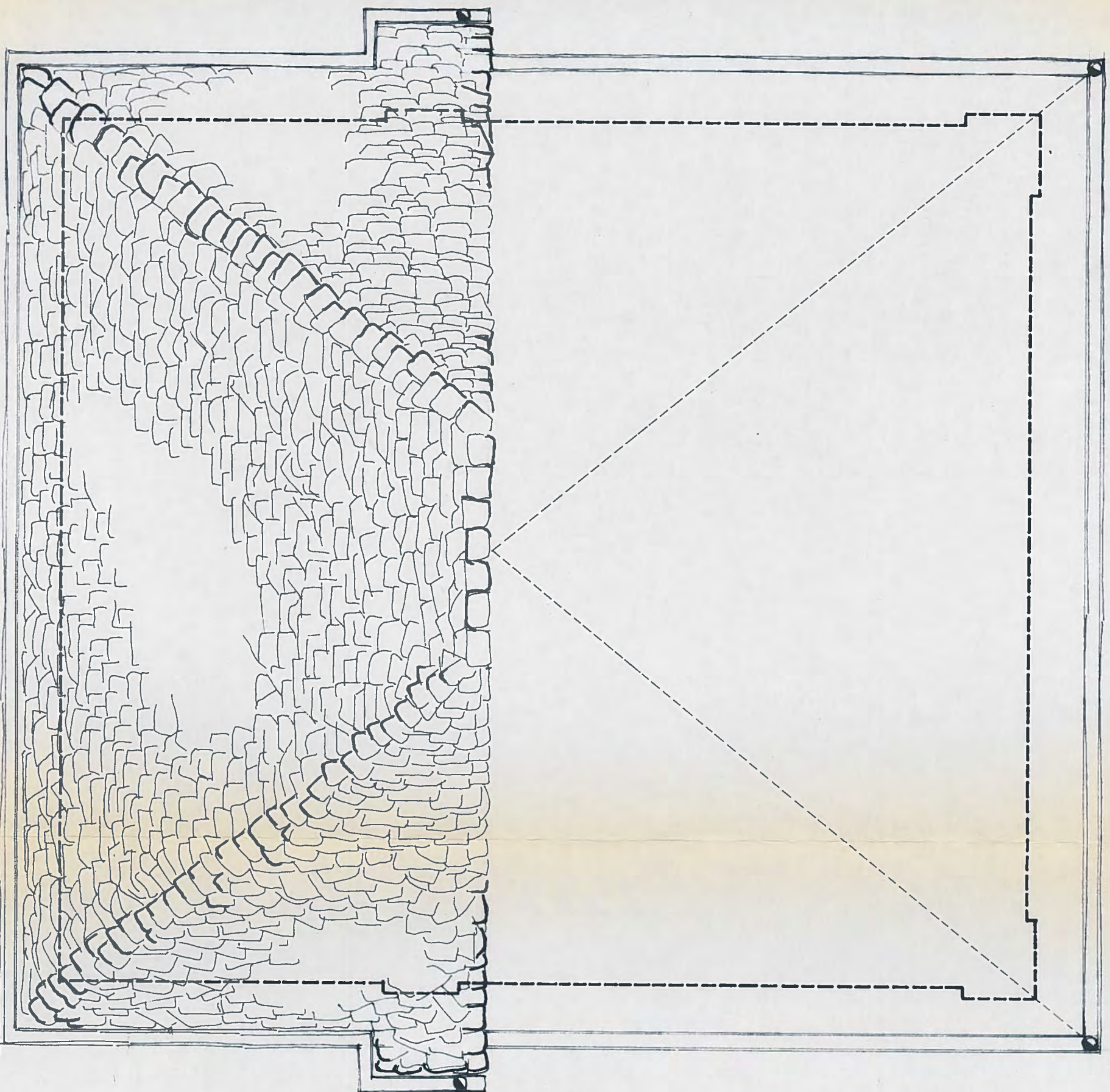
PIANTA DEL TETTO
