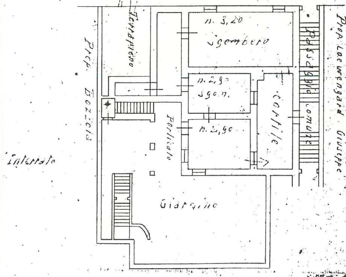
ORTA SAN GIULIO, ISOLA DI SAN GIULIO° Casa ex Steward Pianta scala 1/200
