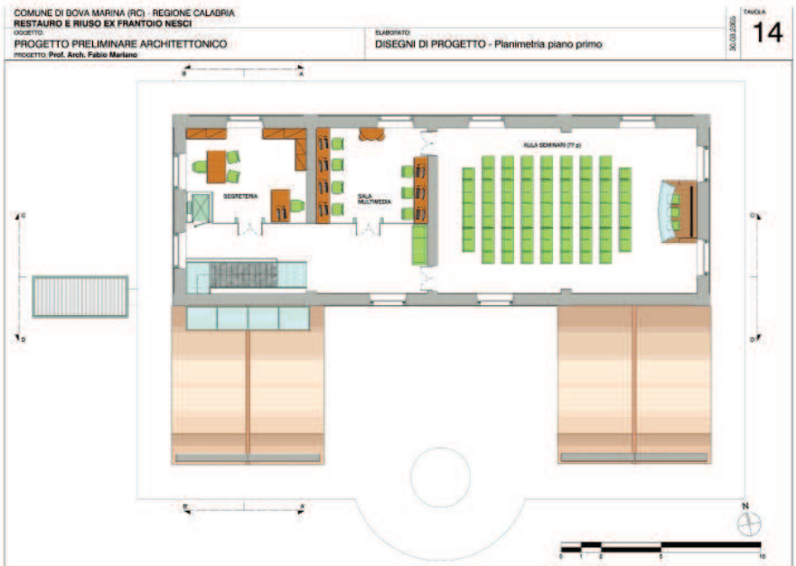
Fig. 13. Progetto di ristrutturazione del Piano primo
