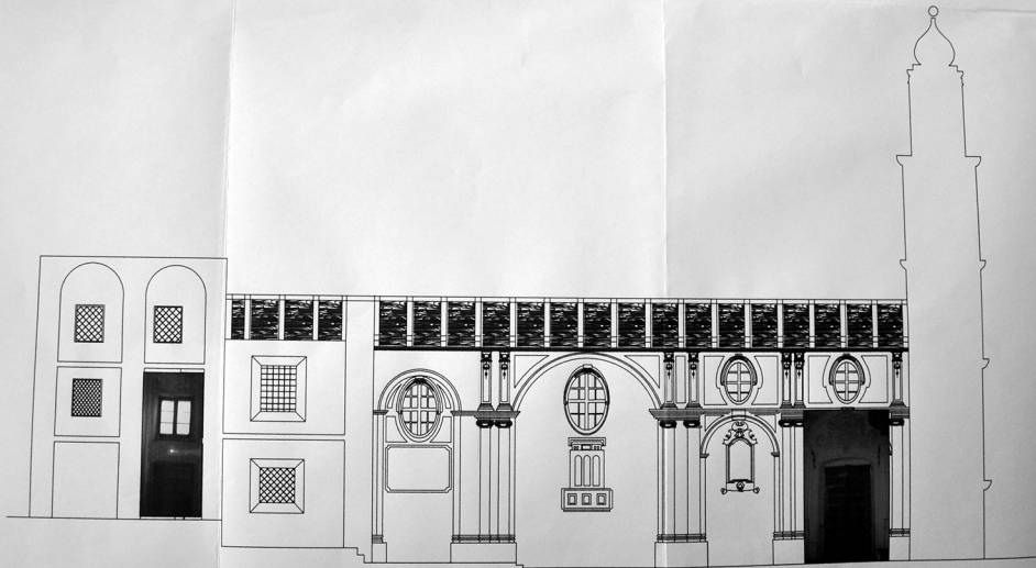
STATO DI FATTO: SEZIONE LONGITUDINALE
