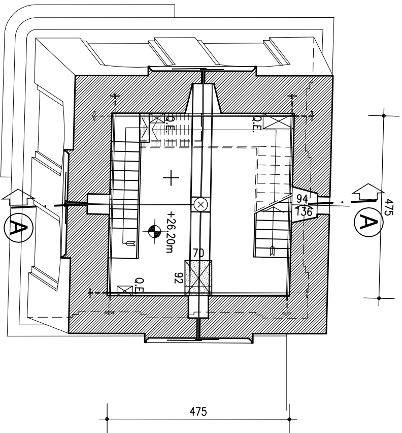
SEZIONE 6-6, scala 1:100
