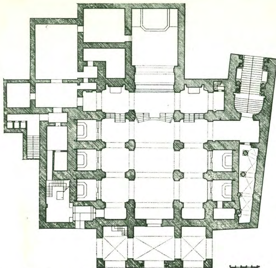
Gaeta. Duomo di S. Erasmo. Pianta.
