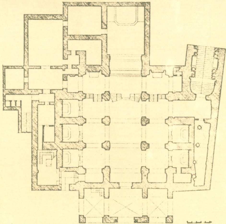
Gaeta. Duomo di S. Erasmo. Pianta.
