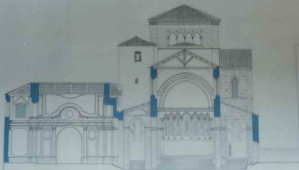
SEZIONE TRASVERSALE sulle Navate -
