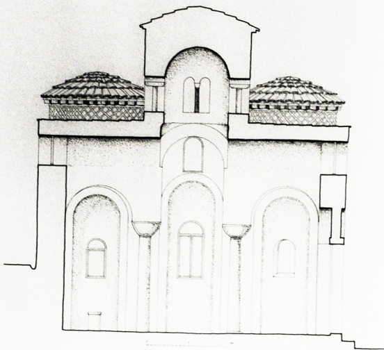
SEZIONE TRASVERSALE
