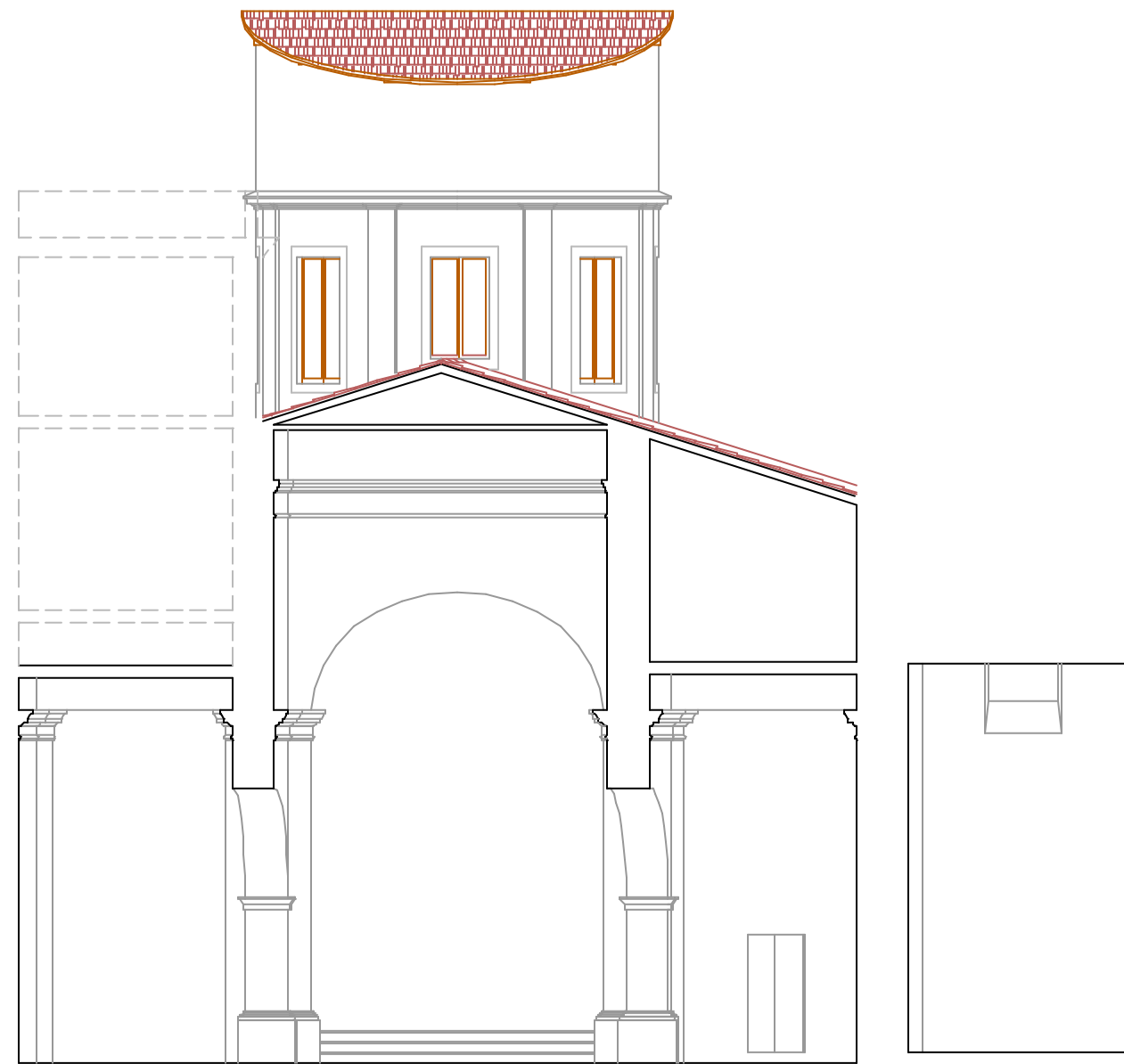
Sezione E - E
