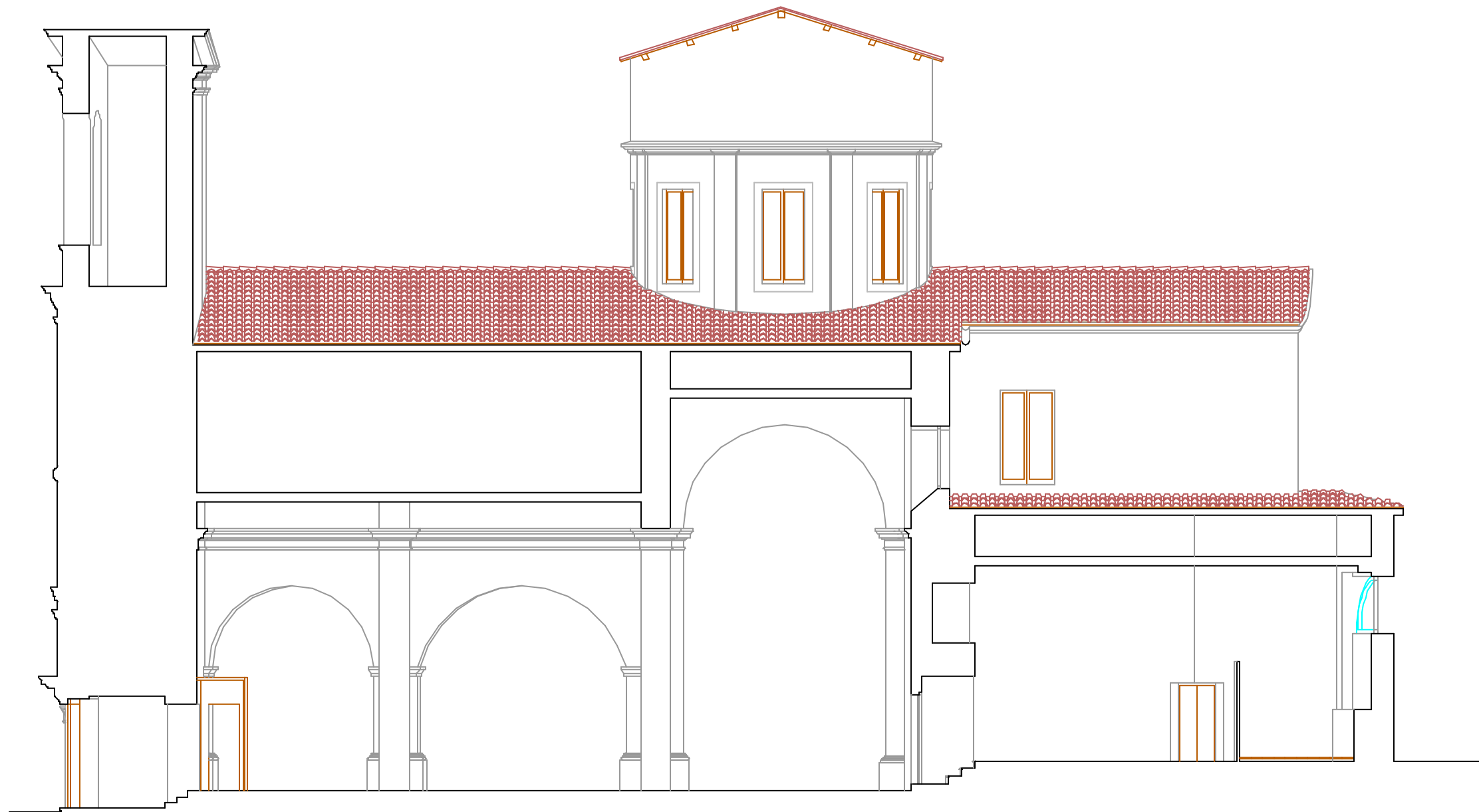
Sezione D - D
