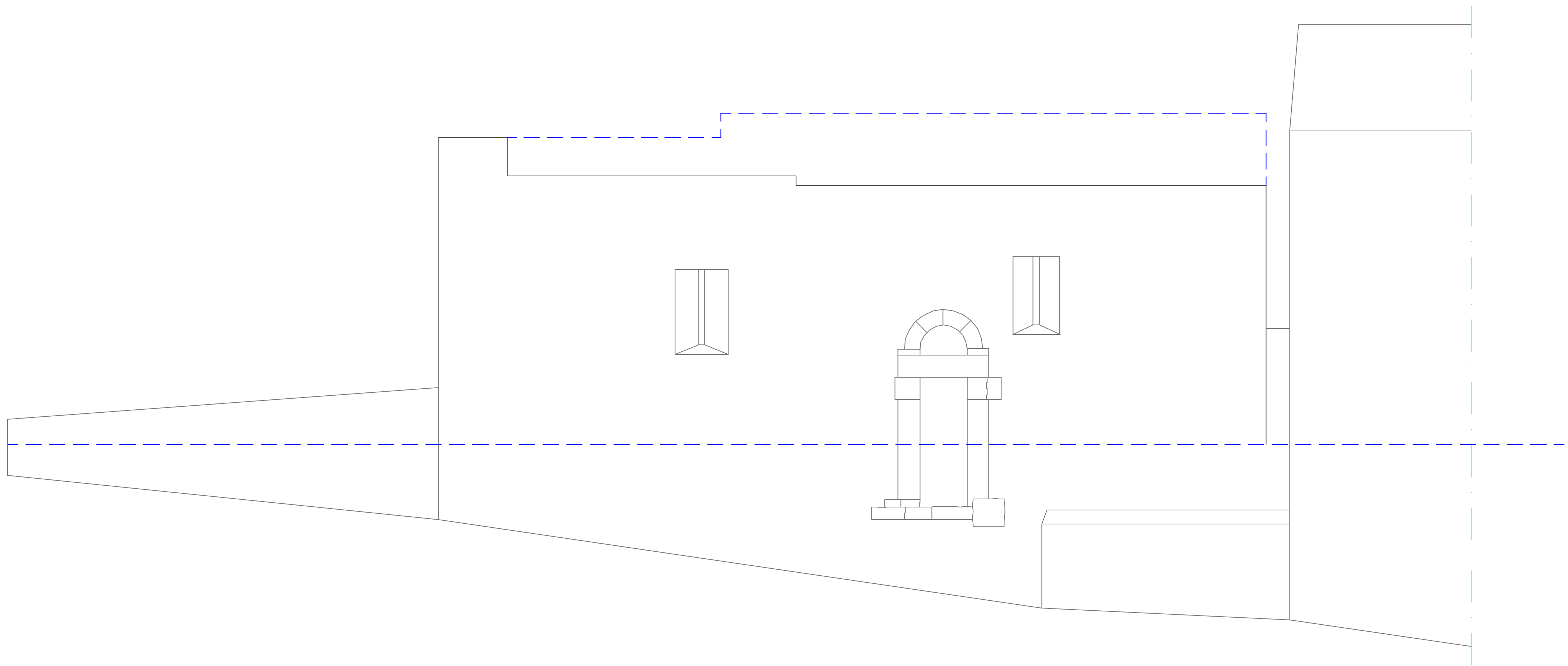
Prospetto Laterale
