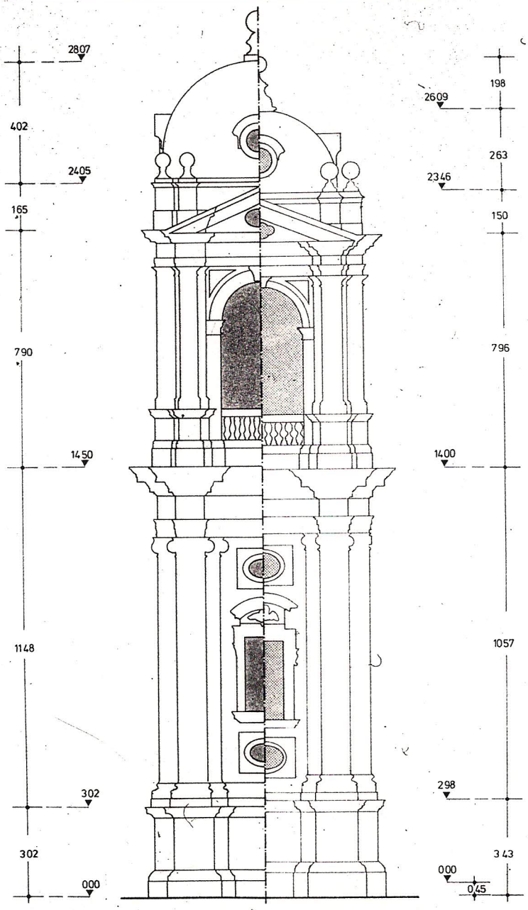
RILIEVO STATO DI FATTO DISEGNO P. COCCAPANI (1864)
