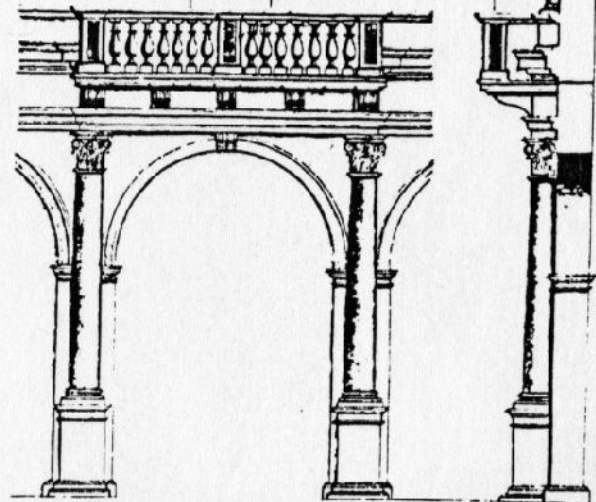
Disegno del nuovo balcone inserito nel piano nobile dell'edificio nel 1787 su progetto del capomastro Giovanni Storni di Milano (B.C.B., Raccolta Gozzadini, cartella 23, n. 43).
