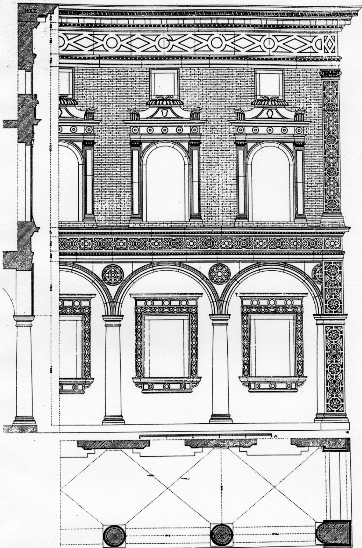
Fig. 48 Palazzo Malvezzi-Campeggi: prospetto parziale (dall'Haupt).
